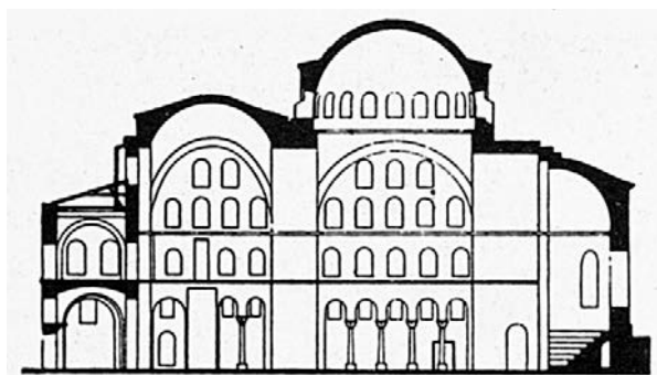
Αγία Ειρήνη (Κωνσταντινούπολη). Σχέδιο κατά Salzenberg.
