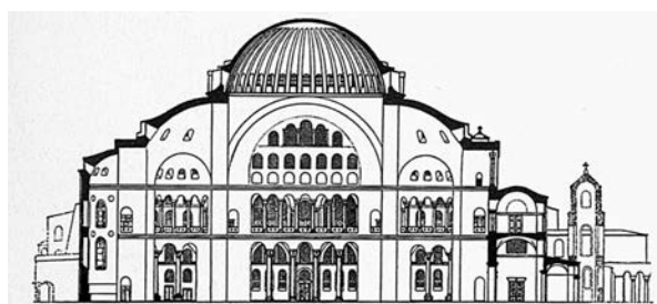
Τομή Αγίας Σοφίας κατά A. M. Schneider.
